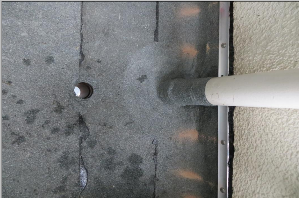
Foto 14 - Randausbildung am Balkonrohr
